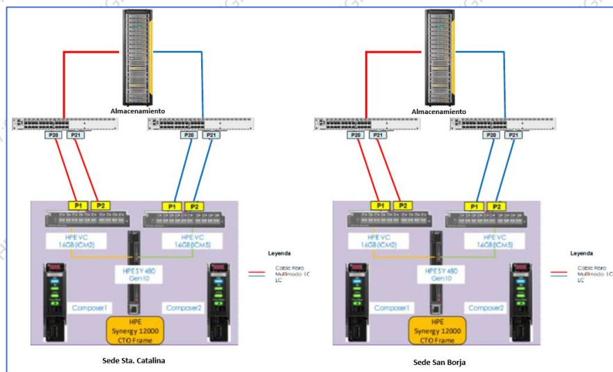
Figura 12. Diagrama servidores de virtualización del RENIEC
