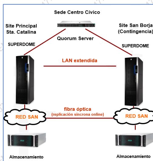
Figura 11. Diagrama servidores misión crítica del RENIEC
